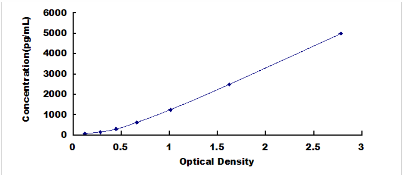
人调节内分泌特异蛋白 18 (RESP18) 检测试剂盒标准曲线
