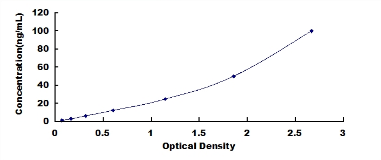
大鼠沉默调节蛋白 2 (SIRT2) 检测试剂盒标准曲线
