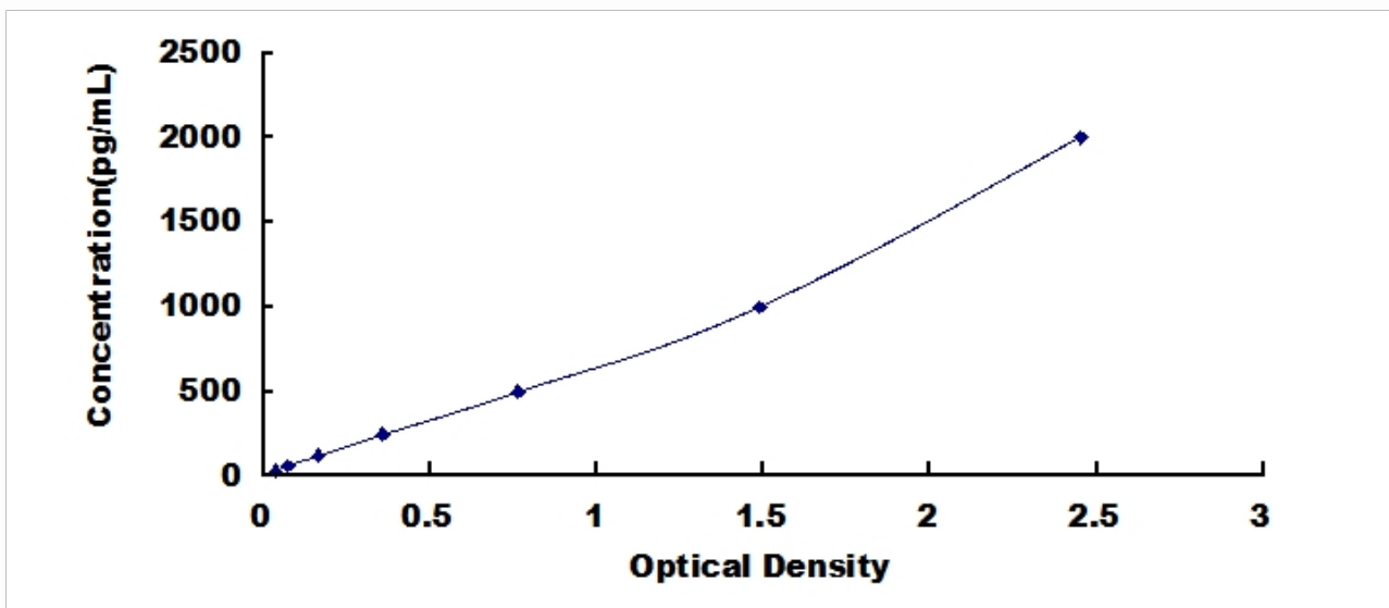
人转化生长因子 \beta 2 (TGF \beta 2) 检测试剂盒标准曲线
