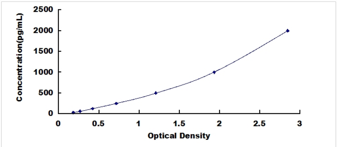
猪转化生长因子 \beta 2 (TGF \beta 2) 检测试剂盒标准曲线
