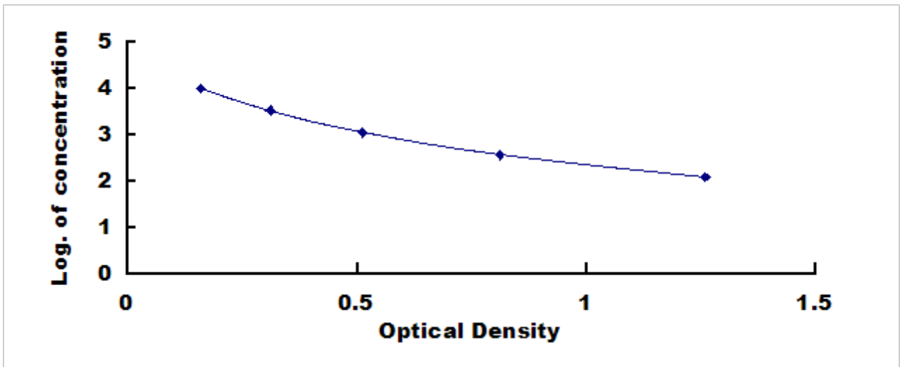
人胰蛋白酶原激活肽 (TAP) 检测试剂盒标准曲线
