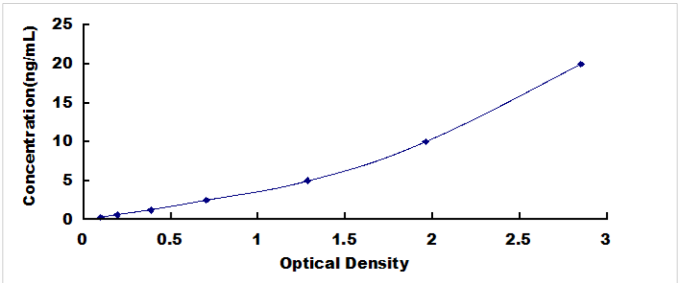
人酪氨酸激酶 2 (Tyk2) 检测试剂盒标准曲线
