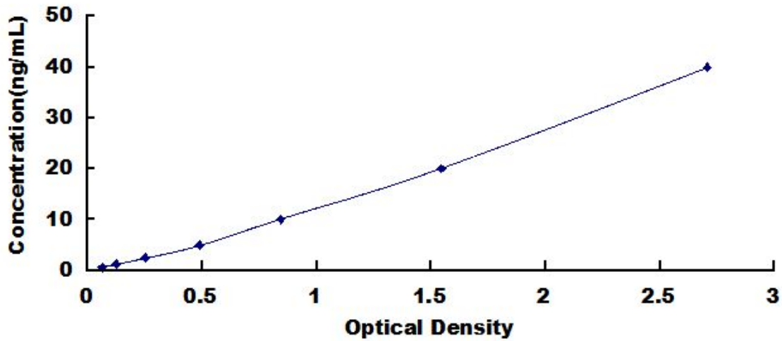
小鼠免疫球蛋白样 EGF 样域酪氨酸激酶 1(Tie1)检测试剂盒标准曲线
