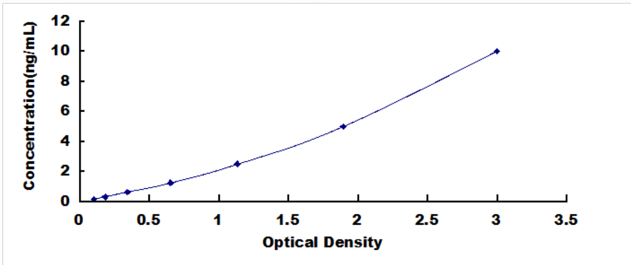
人 UL16 结合蛋白 2 (ULBP2) 检测试剂盒标准曲线
