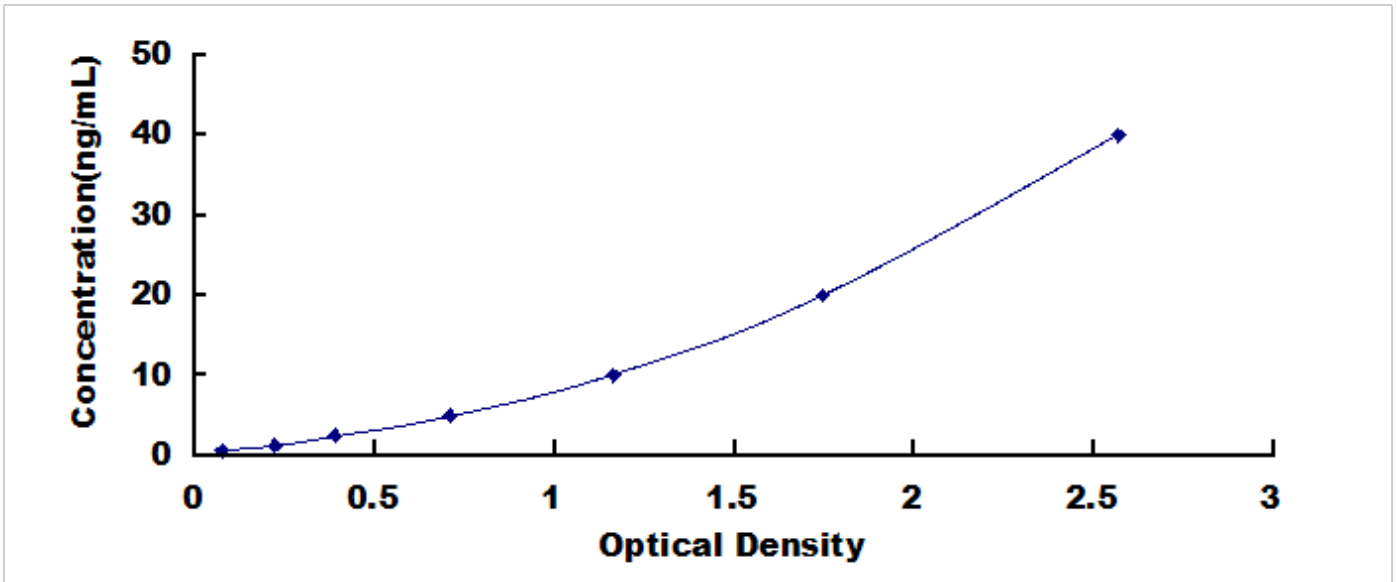
人血管抑制蛋白 1 (VASH1) 检测试剂盒标准曲线
