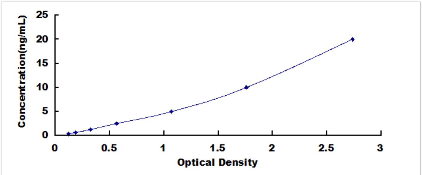
人 Vasorin 蛋白 (VASN) 检测试剂盒标准曲线
