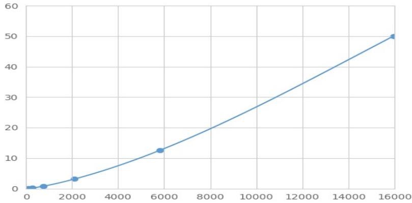
(11-β-羟基类固醇脱氢酶2)检测试剂盒标准曲线
