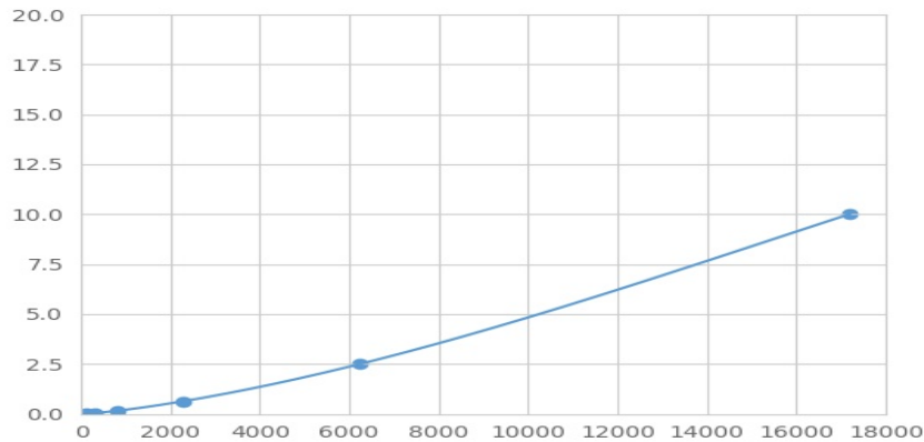
(钠/钾离子转运ATP酶 \alpha 1肽)检测试剂盒标准曲线
