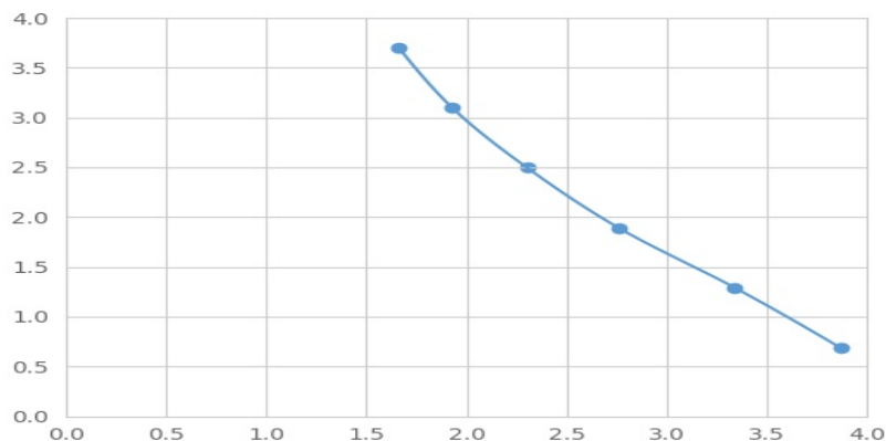
(乙酰肉毒碱)检测试剂盒标准曲线
