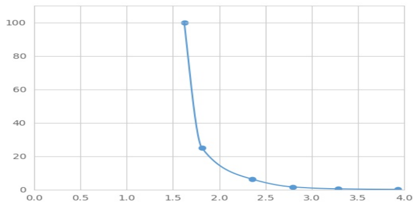
(别孕烯醇酮)检测试剂盒标准曲线
