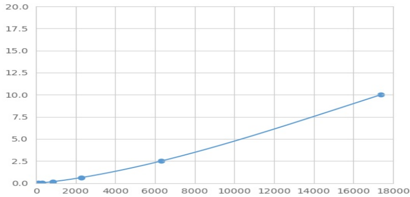
( \alpha -甲基酰基辅酶A消旋酶)检测试剂盒标准曲线
