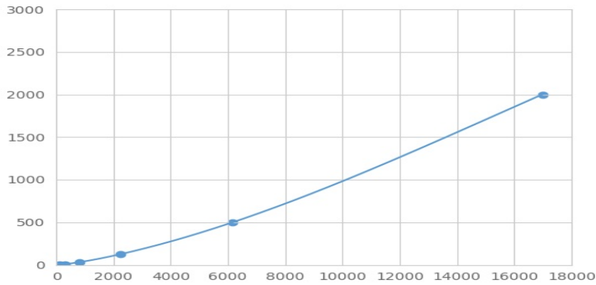
(血管生成素样蛋白2)检测试剂盒标准曲线
