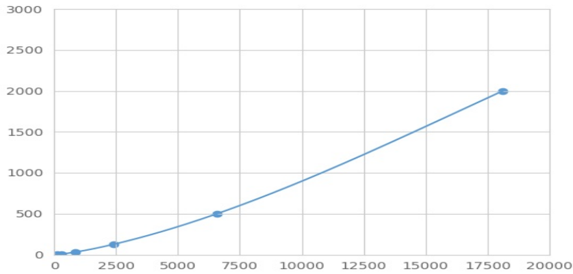
(苯胺素)检测试剂盒标准曲线
