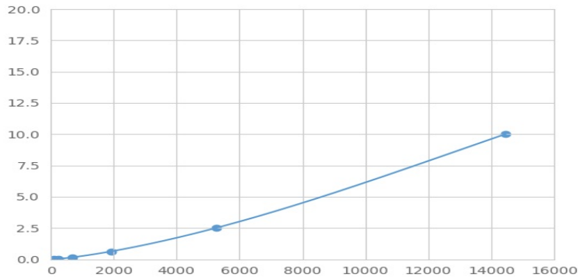
(生物素酰胺酶)检测试剂盒标准曲线
