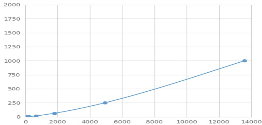
(羧肽酶N1)检测试剂盒标准曲线
