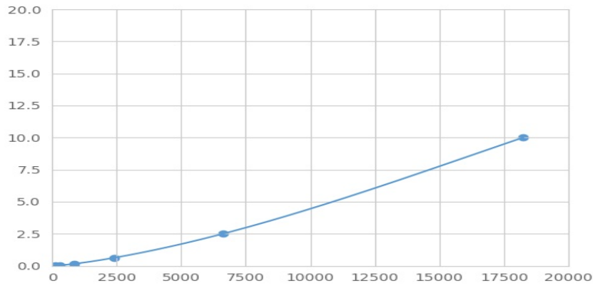
(酪蛋白激酶1δ)检测试剂盒标准曲线
