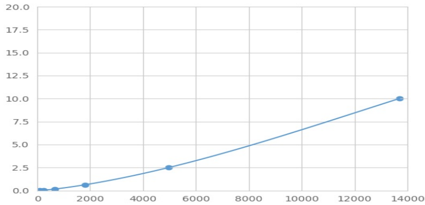
(胆碱乙酰转移酶)检测试剂盒标准曲线
