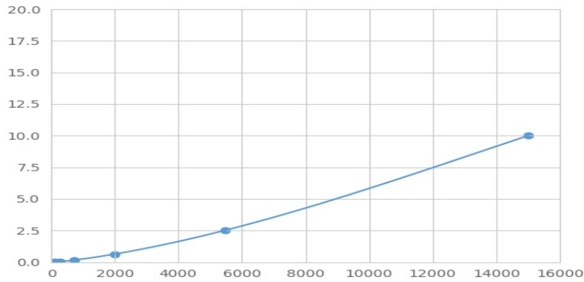
(4号染色体开放阅读框48)检测试剂盒标准曲线
