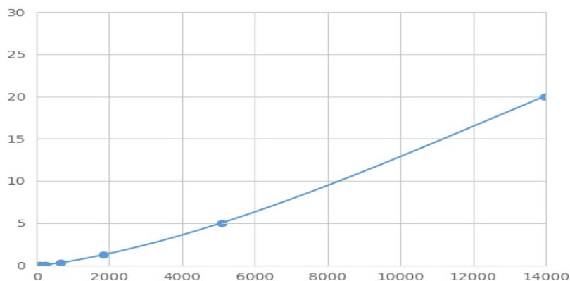
(XII型胶原) 检测试剂盒标准曲线
