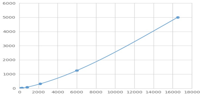
(亲环素B)检测试剂盒标准曲线
