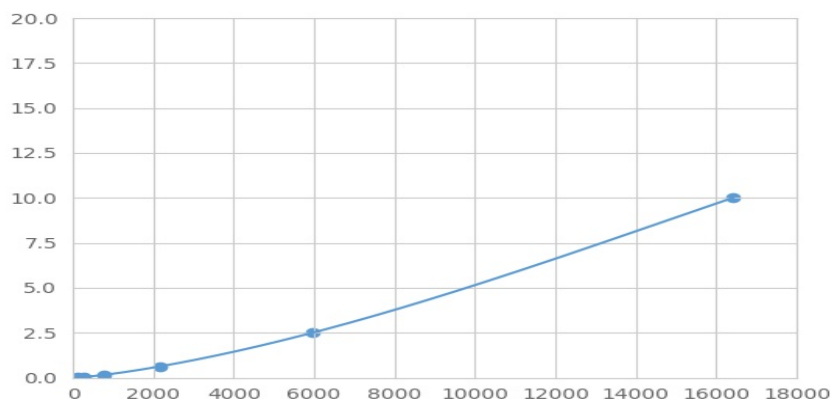
(细胞色素P450家族成员11A1) 检测试剂盒标准曲线
