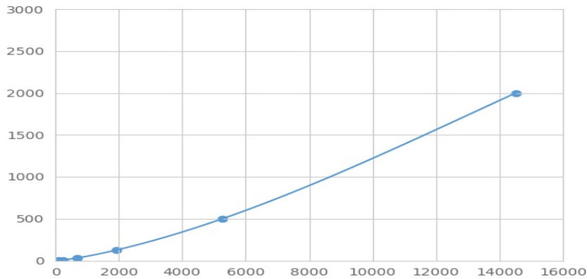
(防御素 α 1B) 检测试剂盒标准曲线
