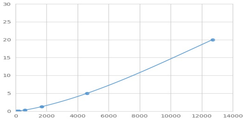
(FK506结合蛋白5)检测试剂盒标准曲线
