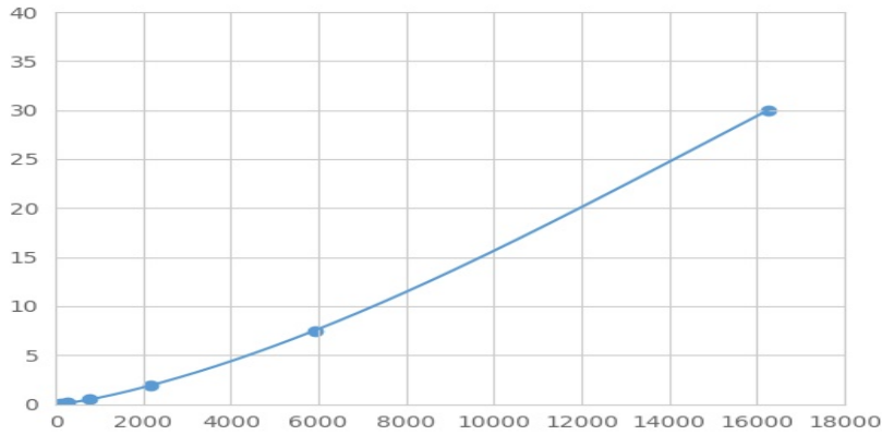
(纤维介素蛋白)检测试剂盒标准曲线
