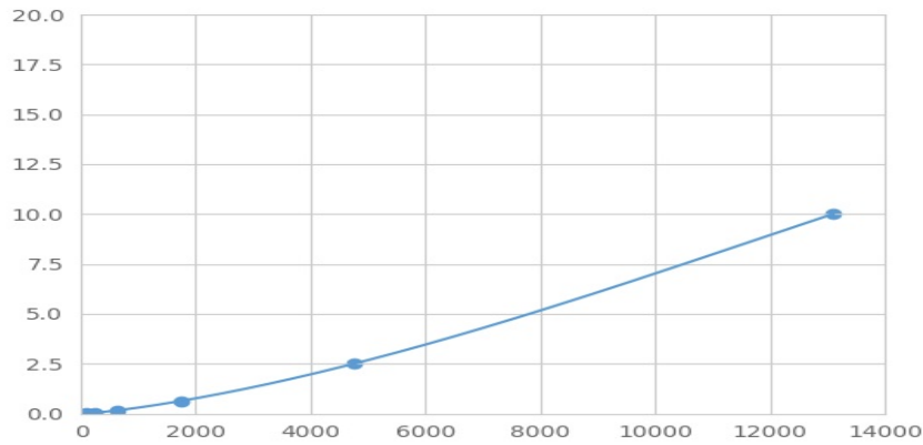
(通用转录因子 II F肽1) 检测试剂盒标准曲线
