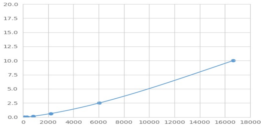
(糖皮质激素受体)检测试剂盒标准曲线
