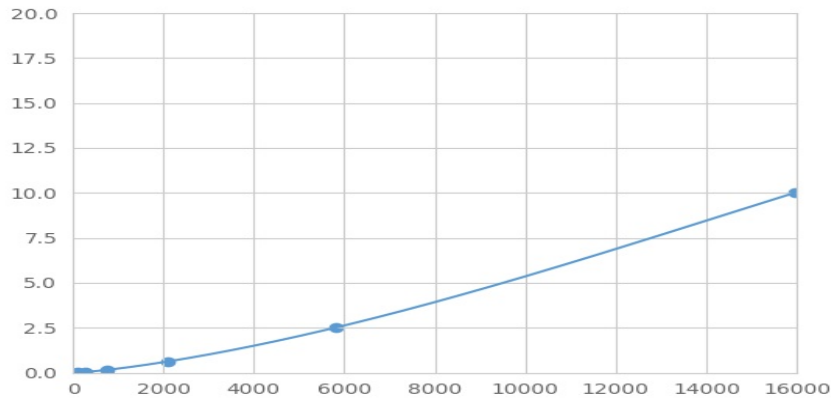
(糖原脱支酶)检测试剂盒标准曲线
