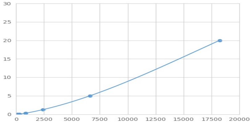
(糖原合酶激酶3 \beta )检测试剂盒标准曲线
