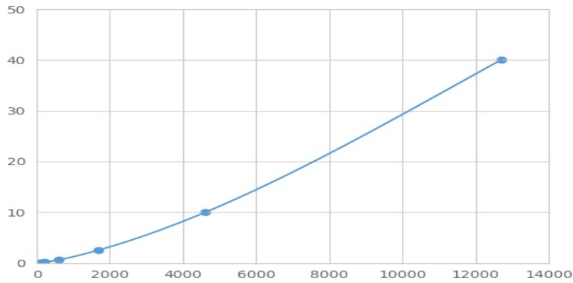
(糖蛋白130)检测试剂盒标准曲线
