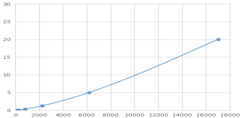
(鸟嘌呤脱氨酶)检测试剂盒标准曲线
