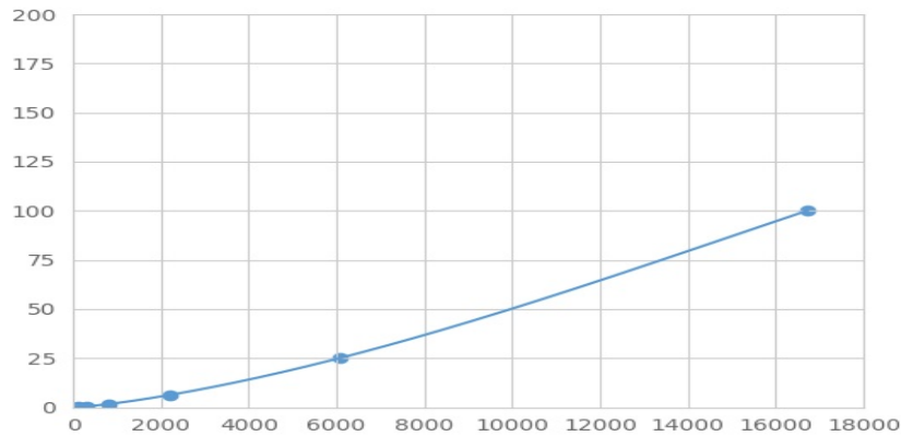
(H2A组蛋白家族成员V)检测试剂盒标准曲线
