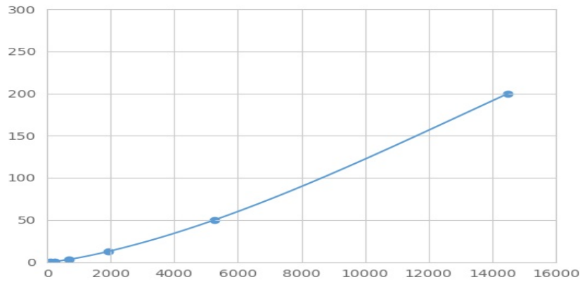
(高分子量激肽原)检测试剂盒标准曲线
