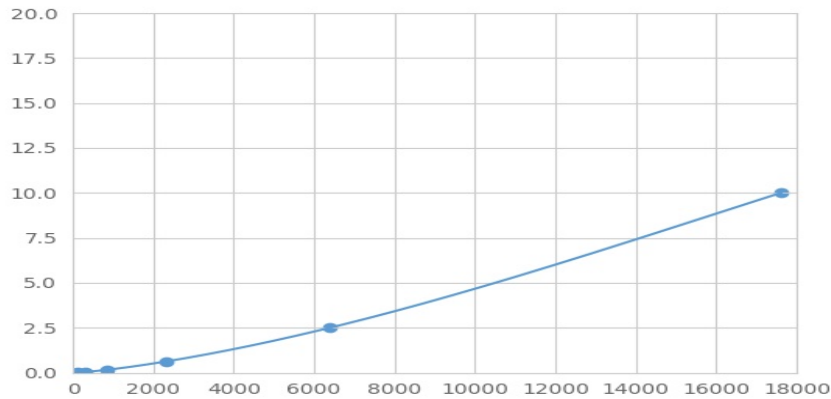
(组蛋白脱乙酰基酶1)检测试剂盒标准曲线
