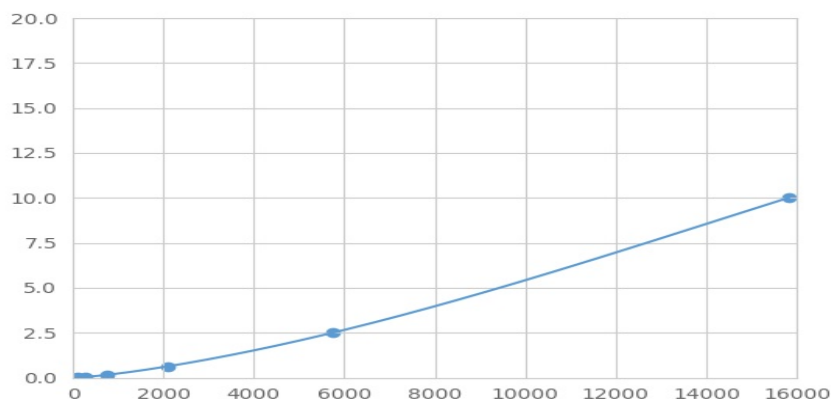
(羟甲基戊二酰辅酶A合酶)检测试剂盒标准曲线
