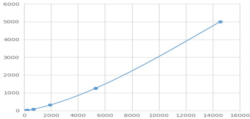
(核因子 \kappa B抑制因子 \zeta )检测试剂盒标准曲线
