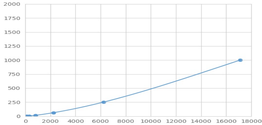
(干扰素 α 2) 检测试剂盒标准曲线
