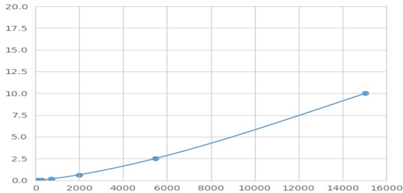
(白介素1受体辅助蛋白)检测试剂盒标准曲线
