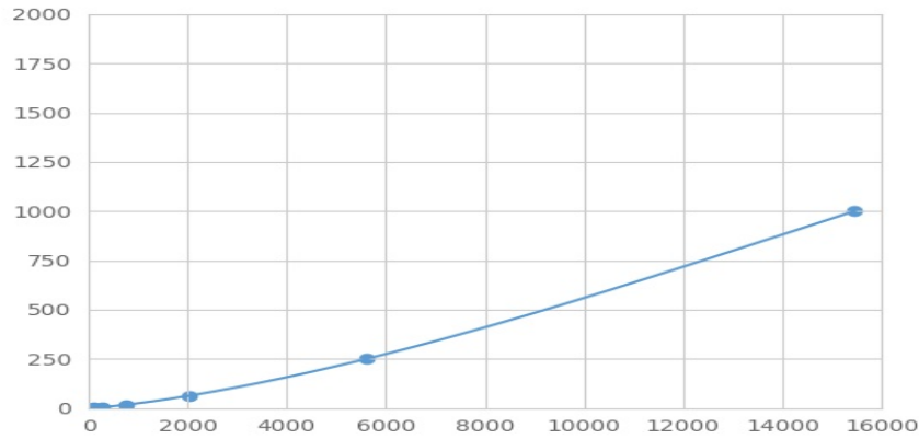
(白介素15)检测试剂盒标准曲线
