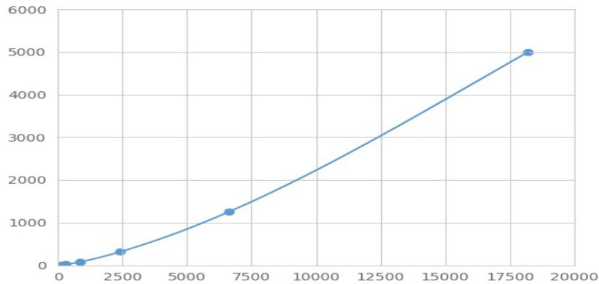
(亮氨酸脯氨酸富集多糖1)检测试剂盒标准曲线
