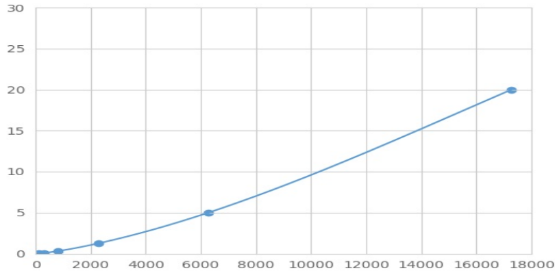
(含亮氨酸丰富重复蛋白15)检测试剂盒标准曲线
