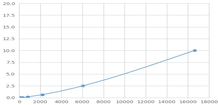
(基质金属蛋白酶28)检测试剂盒标准曲线
