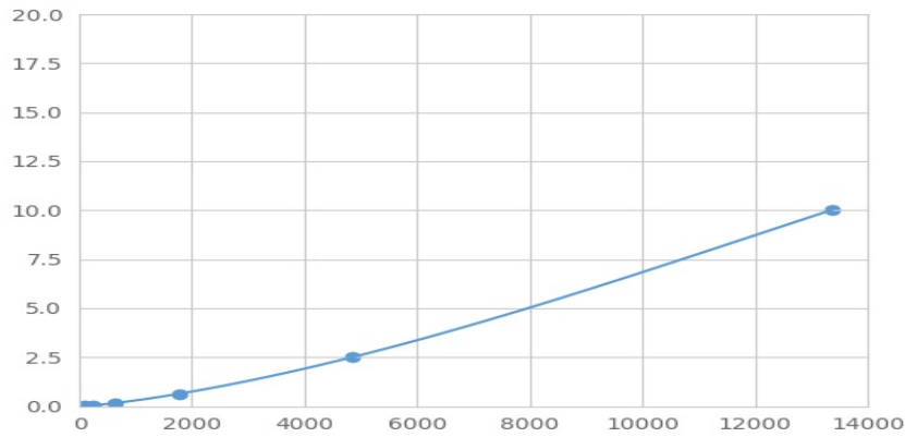
(神经细胞粘附分子)检测试剂盒标准曲线
