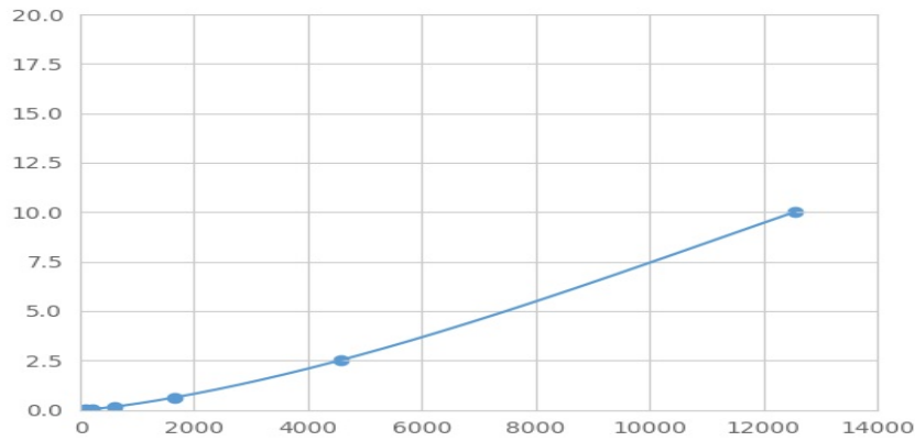
(核因子 κ B)检测试剂盒标准曲线
