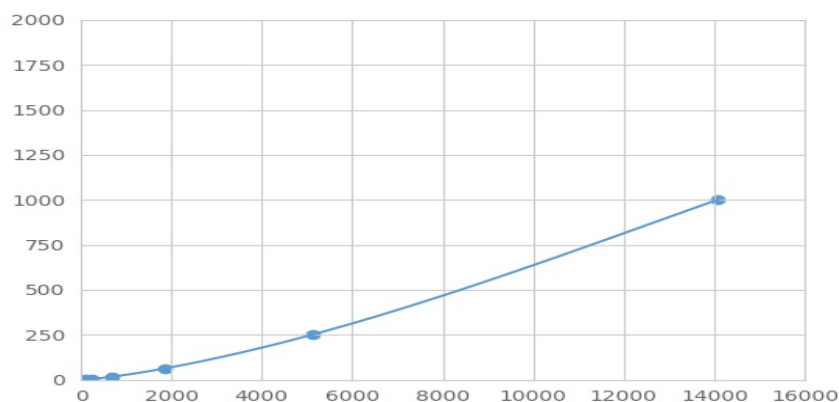
(氧化低密度脂蛋白)检测试剂盒标准曲线
