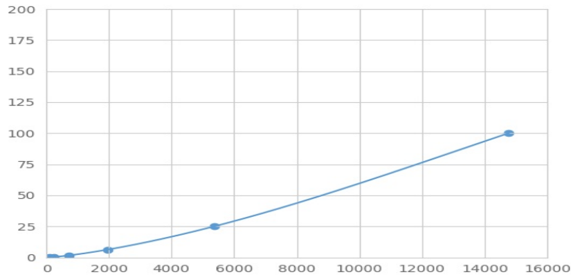
(对氧磷酶3)检测试剂盒标准曲线
