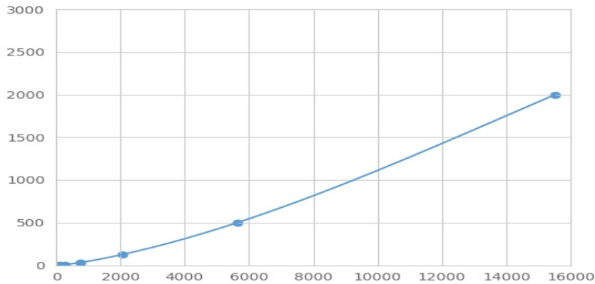
(旁血小板溶蛋白)检测试剂盒标准曲线
